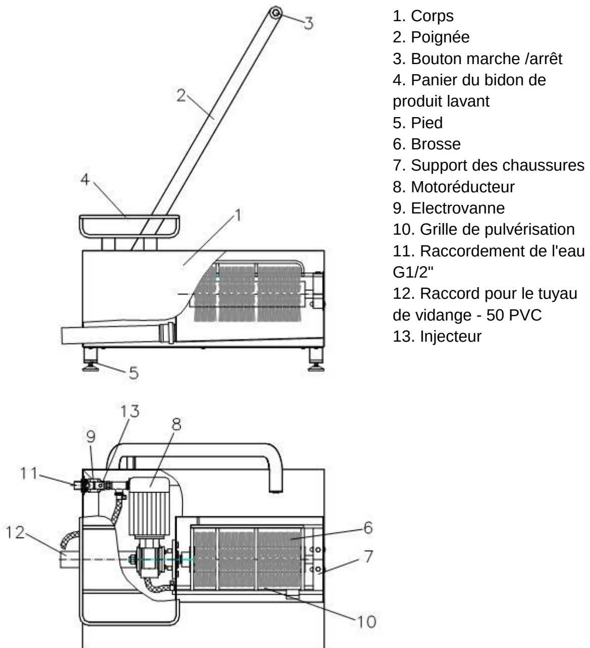
Figure 1. Vue éclatée
