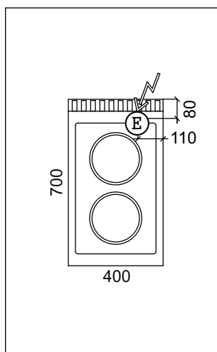
Fig. 18 Cuisinière 2 plaques
