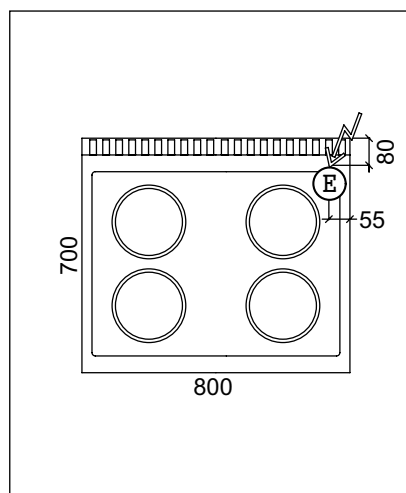
Fig. 19 Cuisinière 4 plaques
