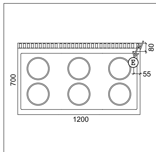
Fig. 20 Cuisinière 6 plaques
