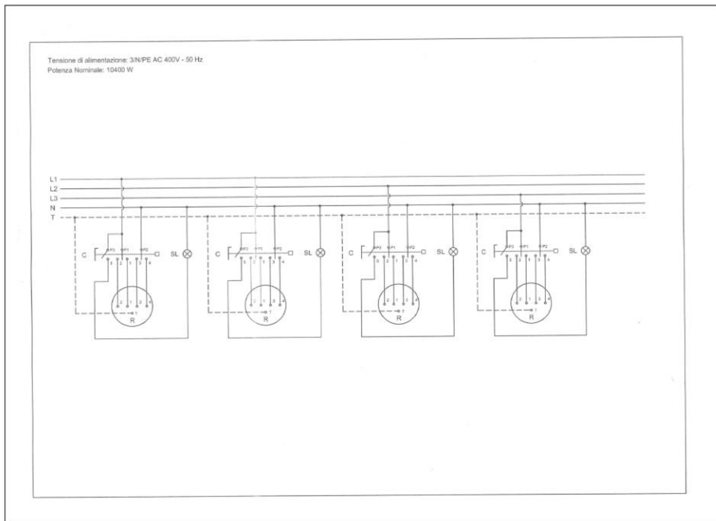
Fig. 25 Schéma électrique 1 - Appareil
