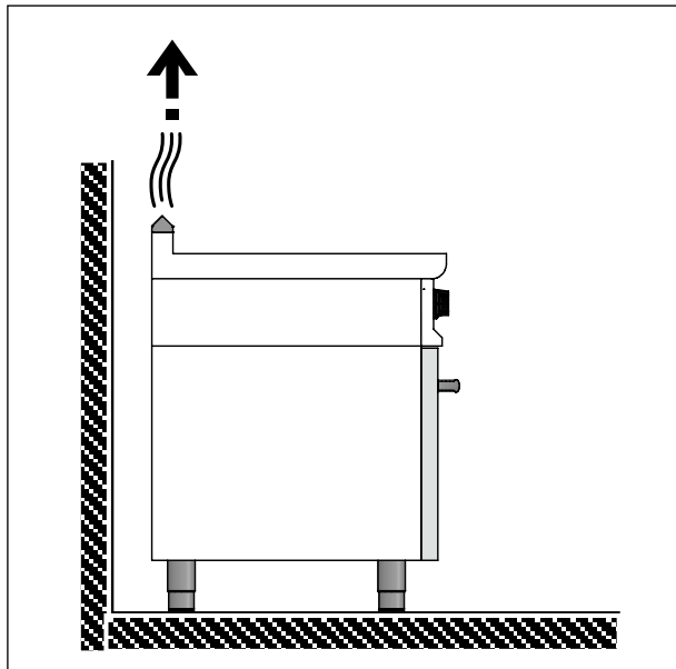
Fig. 22 Échappement chaleur
