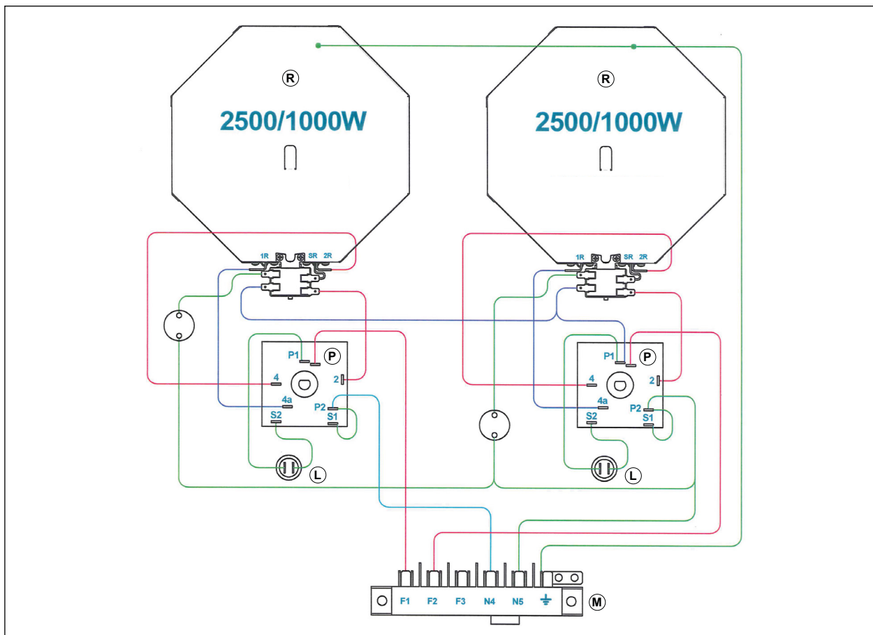
Fig. 24 Schéma électrique 2 résistances
