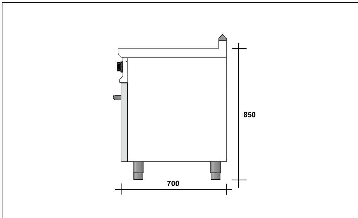
Fig. 16 Dimensions de la cuisinière plan en vitrocéramique
