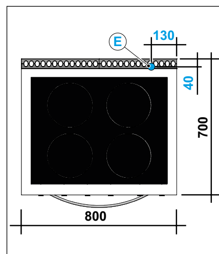
Fig. 19 Cuisinière avec four
