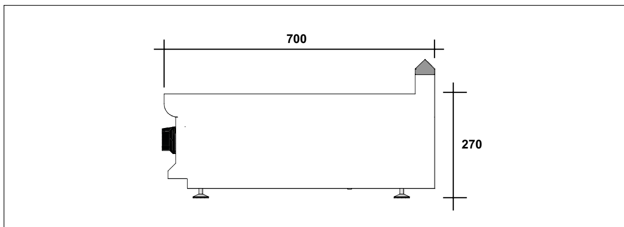
Fig. 13 Dimensions de la cuisinière de comptoir en vitrocéramique
