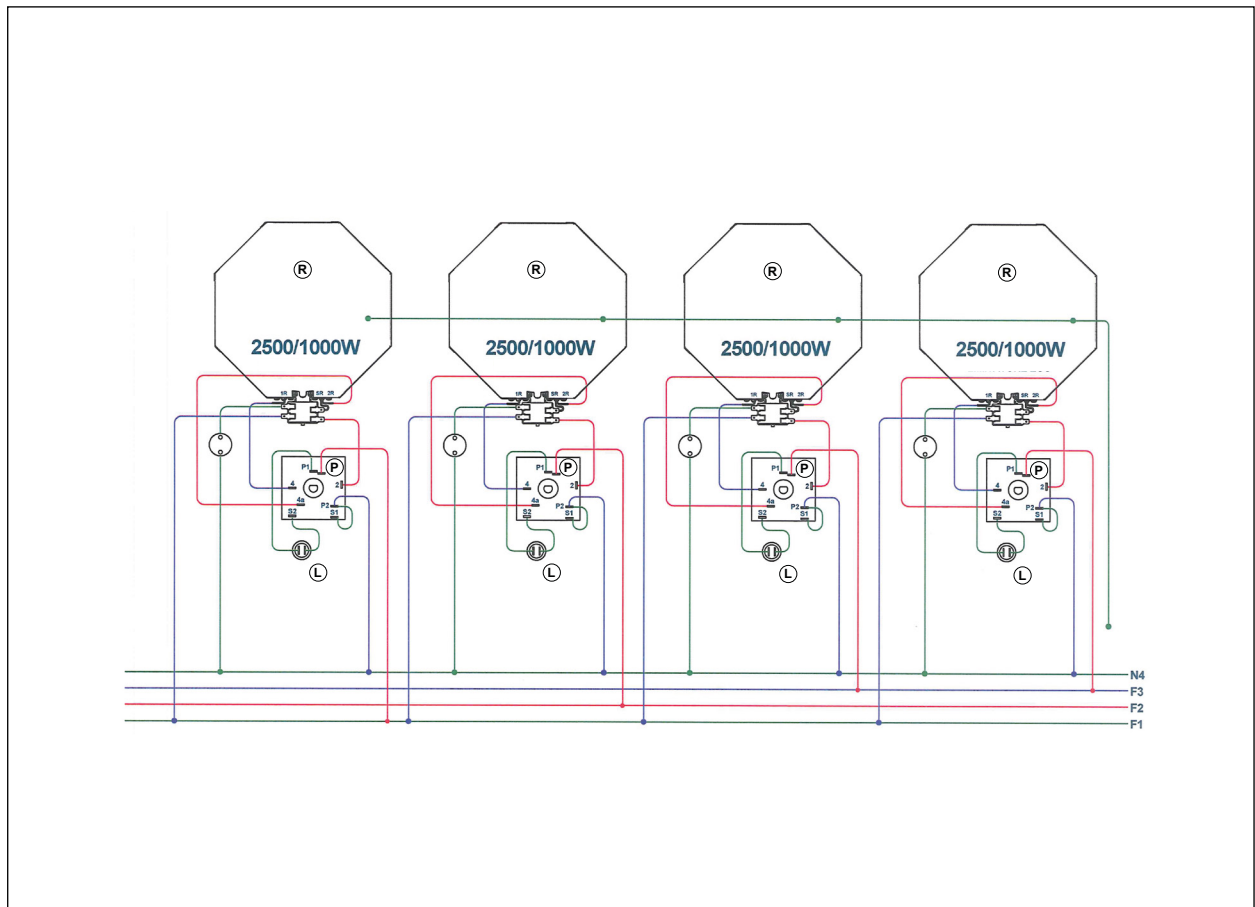
Fig. 25 Schéma électrique 4 résistances
