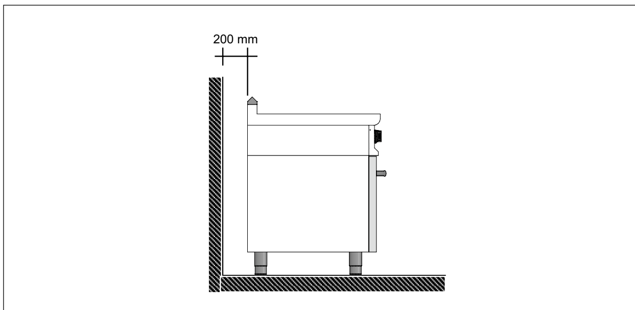
Fig. 20 Distance minimum de parois inflammables
