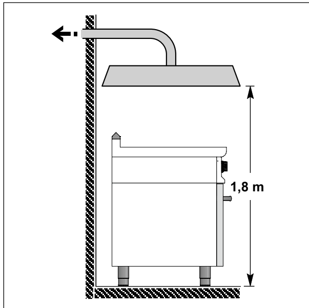
Fig. 23 Échappement à travers une hotte
