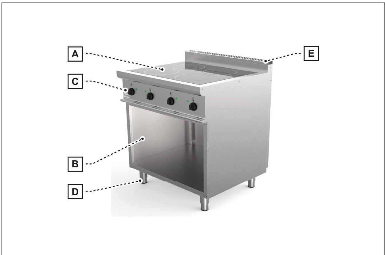
Fig. 4 Parties principales de l'appareil
