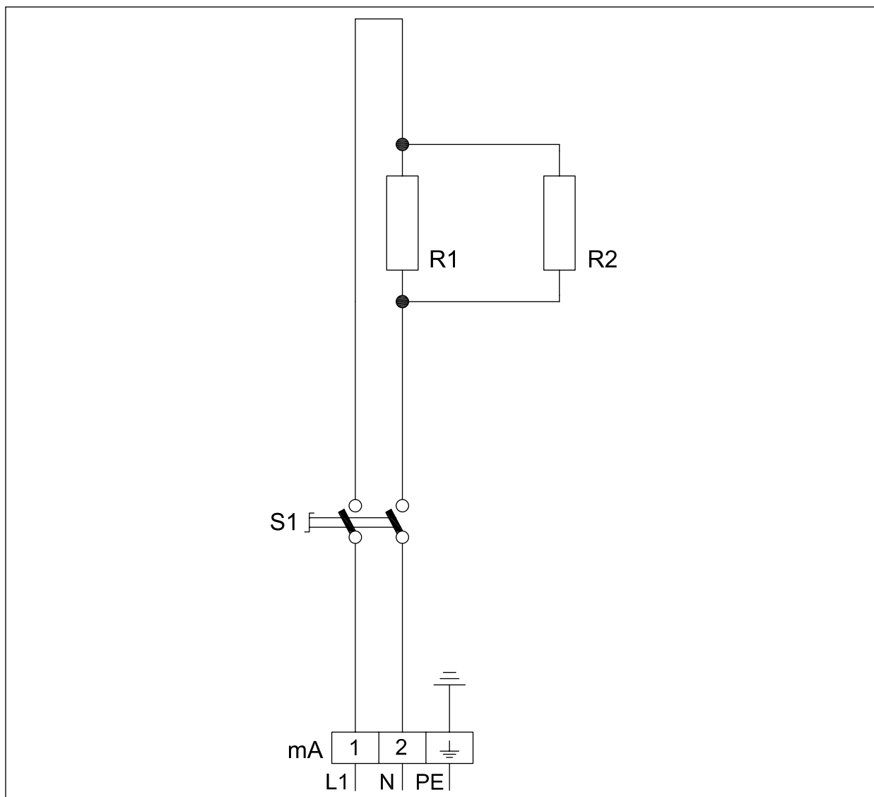
Fig. 18 Schéma électrique
