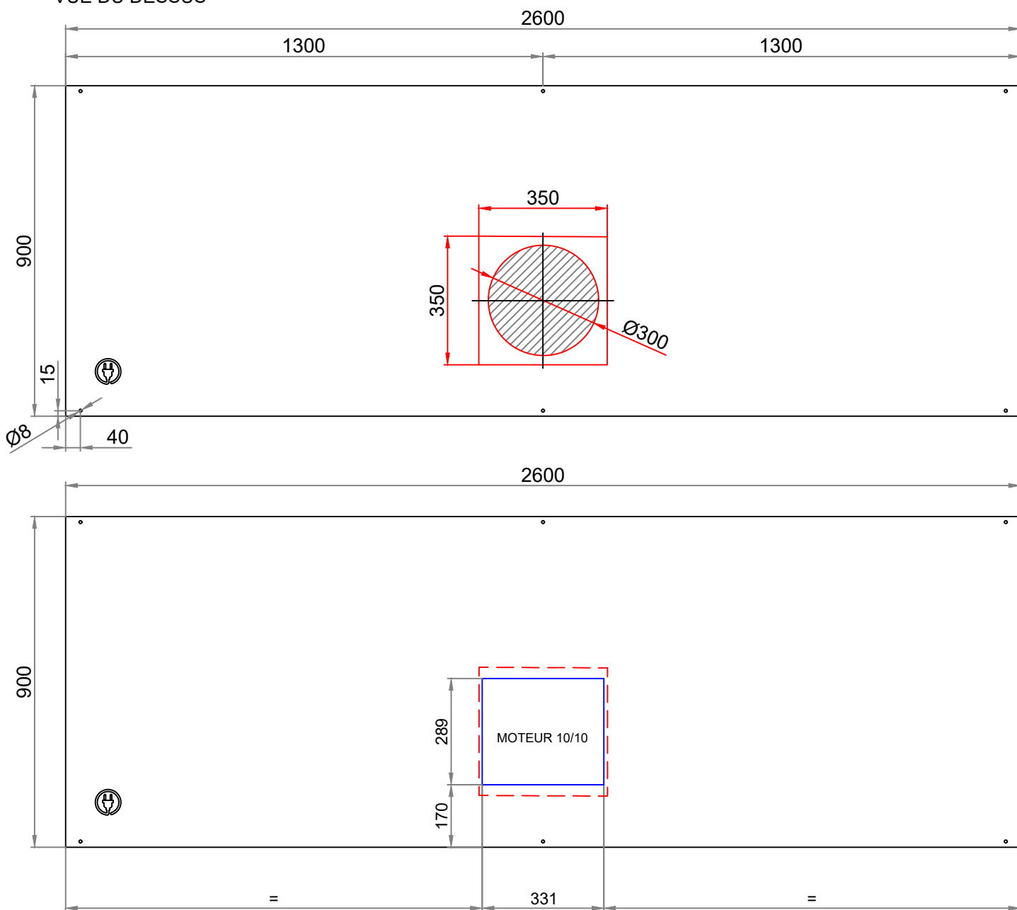
VUE DU DESSUS
