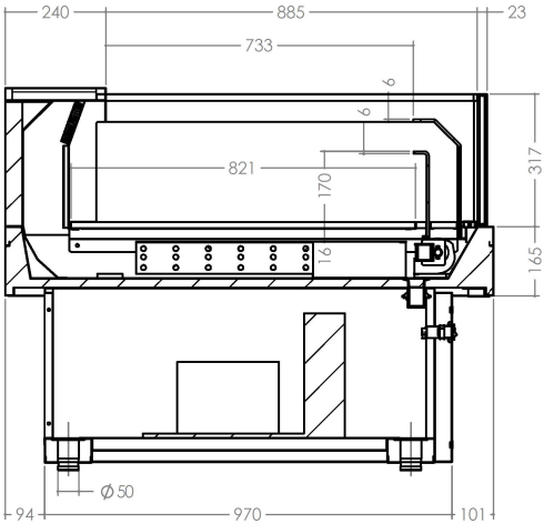
coupe A-A
