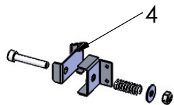
DETTAGLIO H kit bloccaggio vetro interno
