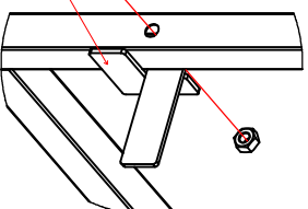
Détail A 1 : 5
