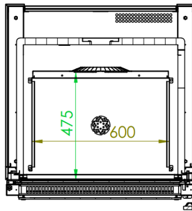
SEZIONE E-E
