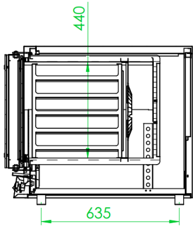
SEZIONE D-D
